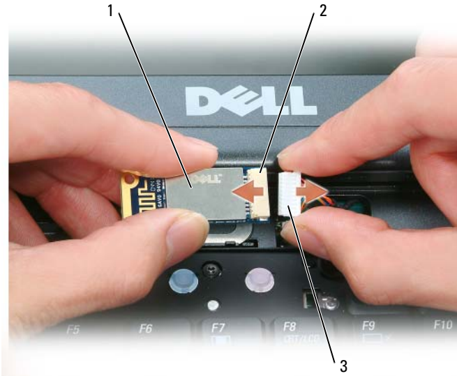
1 카드 2 카드 커넥터 3 케이블 커넥터
