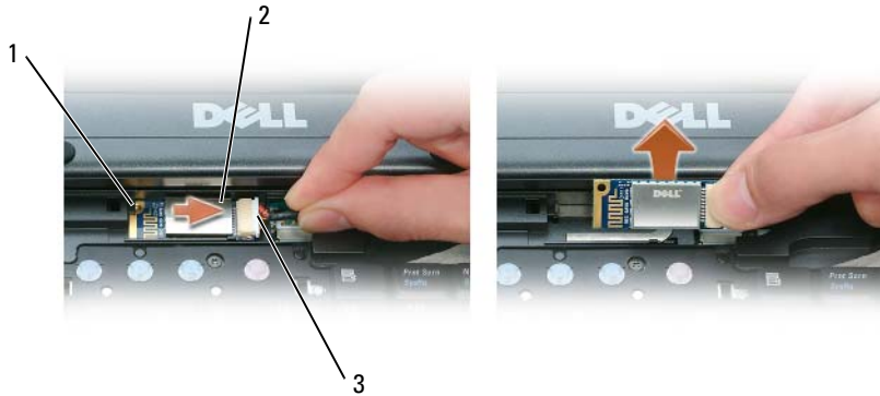
1 금속 탭 2 카드 3 케이블 커넥터
